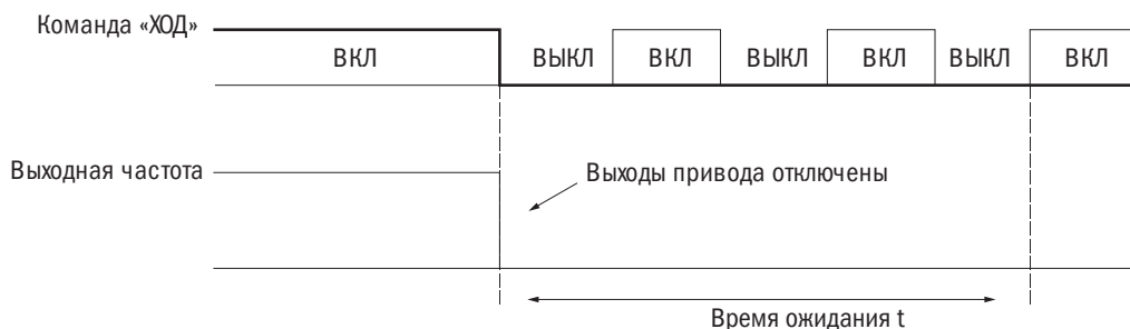
Рис. 6.8. Работа по инерции до остановки с таймером
