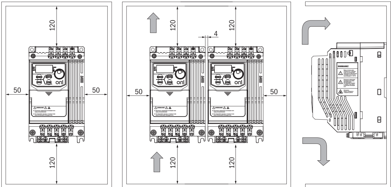
Рис. 3.2. Установка преобразователей
